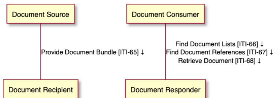
Slika 1 – Komponente i transakcije integracijskog profila IHE MHD
